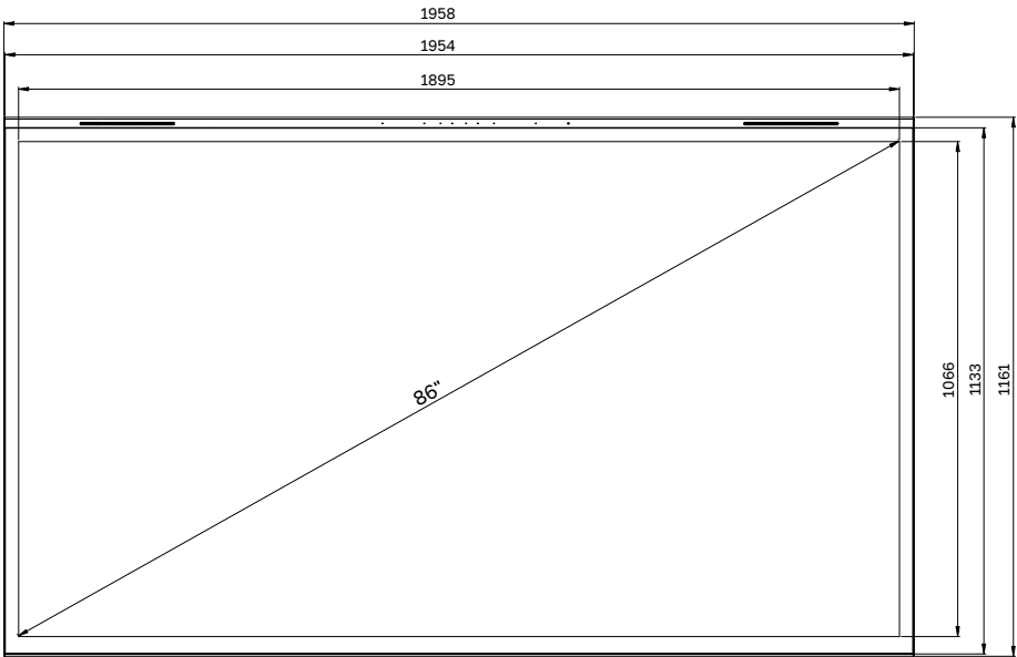
СХЕМА ПАНЕЛИ (ВИД СПЕРЕДИ)
