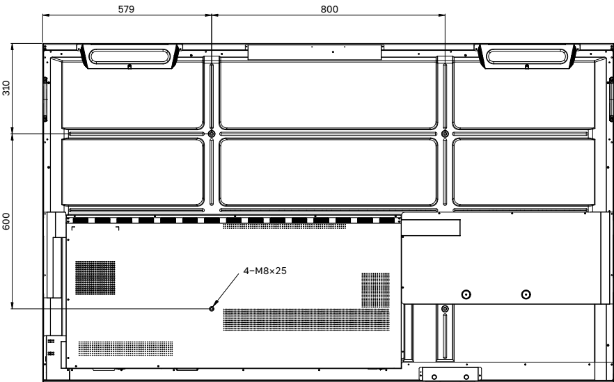
СХЕМА ПАНЕЛИ (ВИД СЗАДИ)
